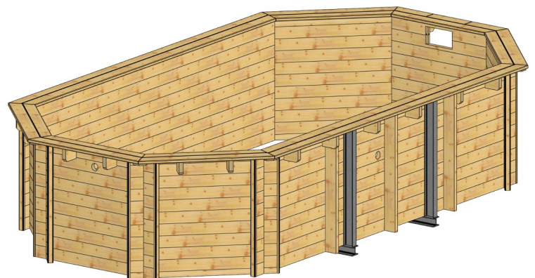
Image de l'ossature complètement montée
